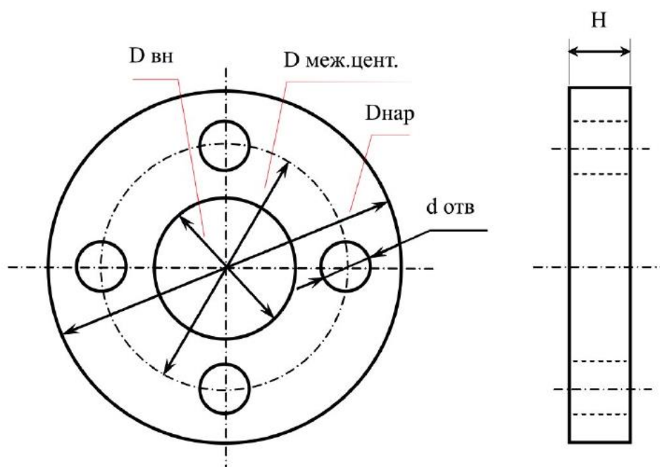
Рис. 5 Эскиз фланца
